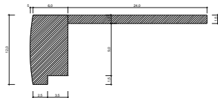
PROFIL PIONOWY - BOCZNY RAMY DREWNIANEJ OSEONY GRZEJNIKOEJ 1 : 2
